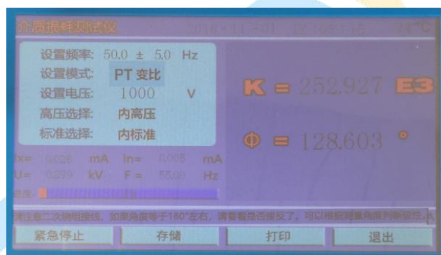
图十八 变比测试结果
