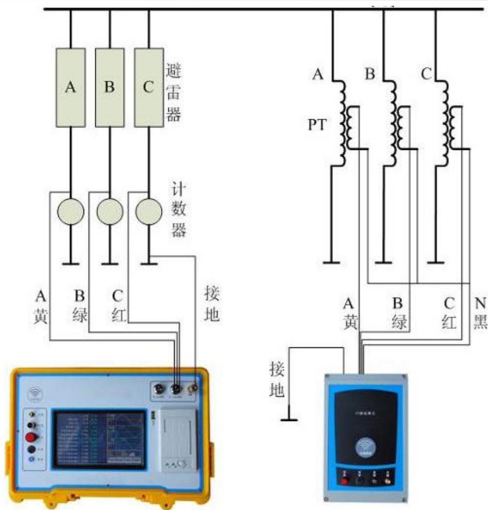
图 2 测试线接线示意图
